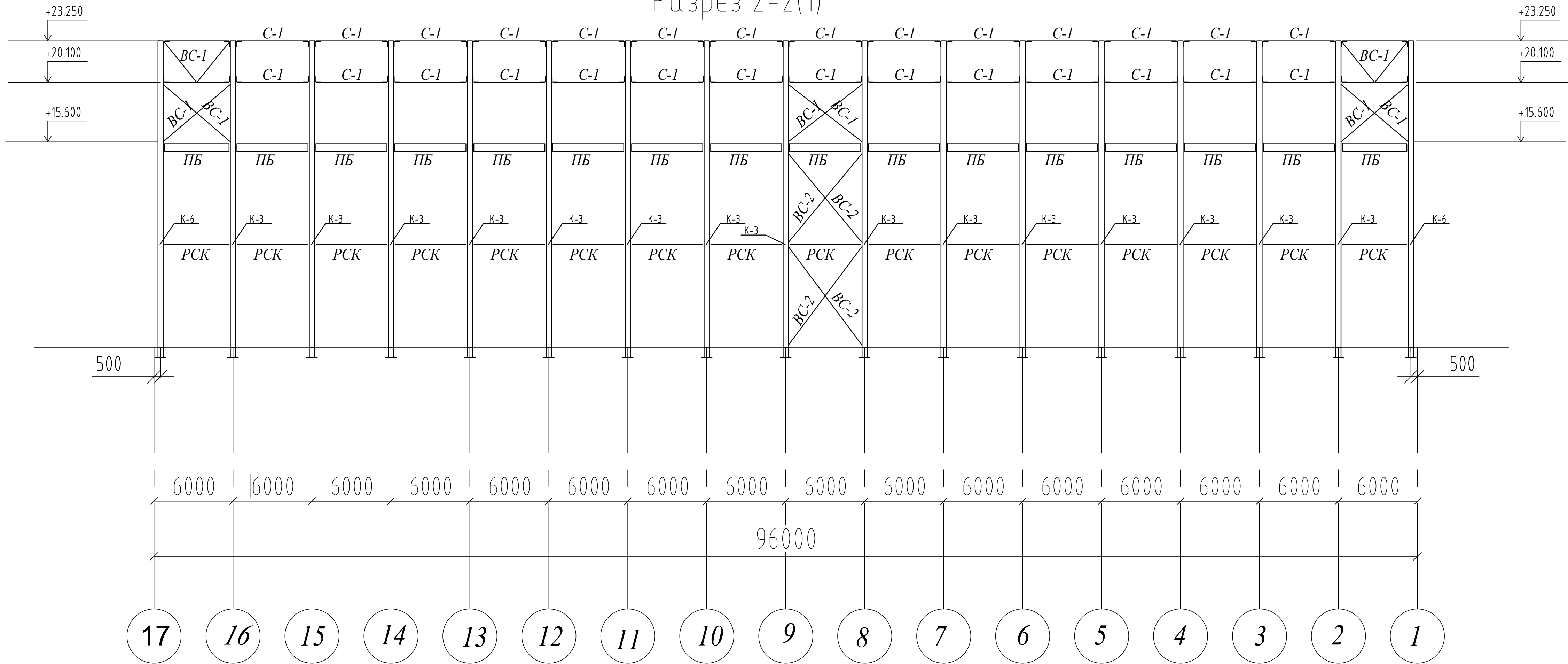
Разрез 2-2(1)
