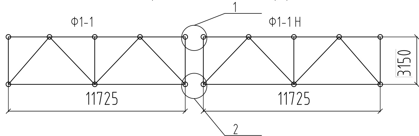
Схема отправочных элементов фермы Ф-1
