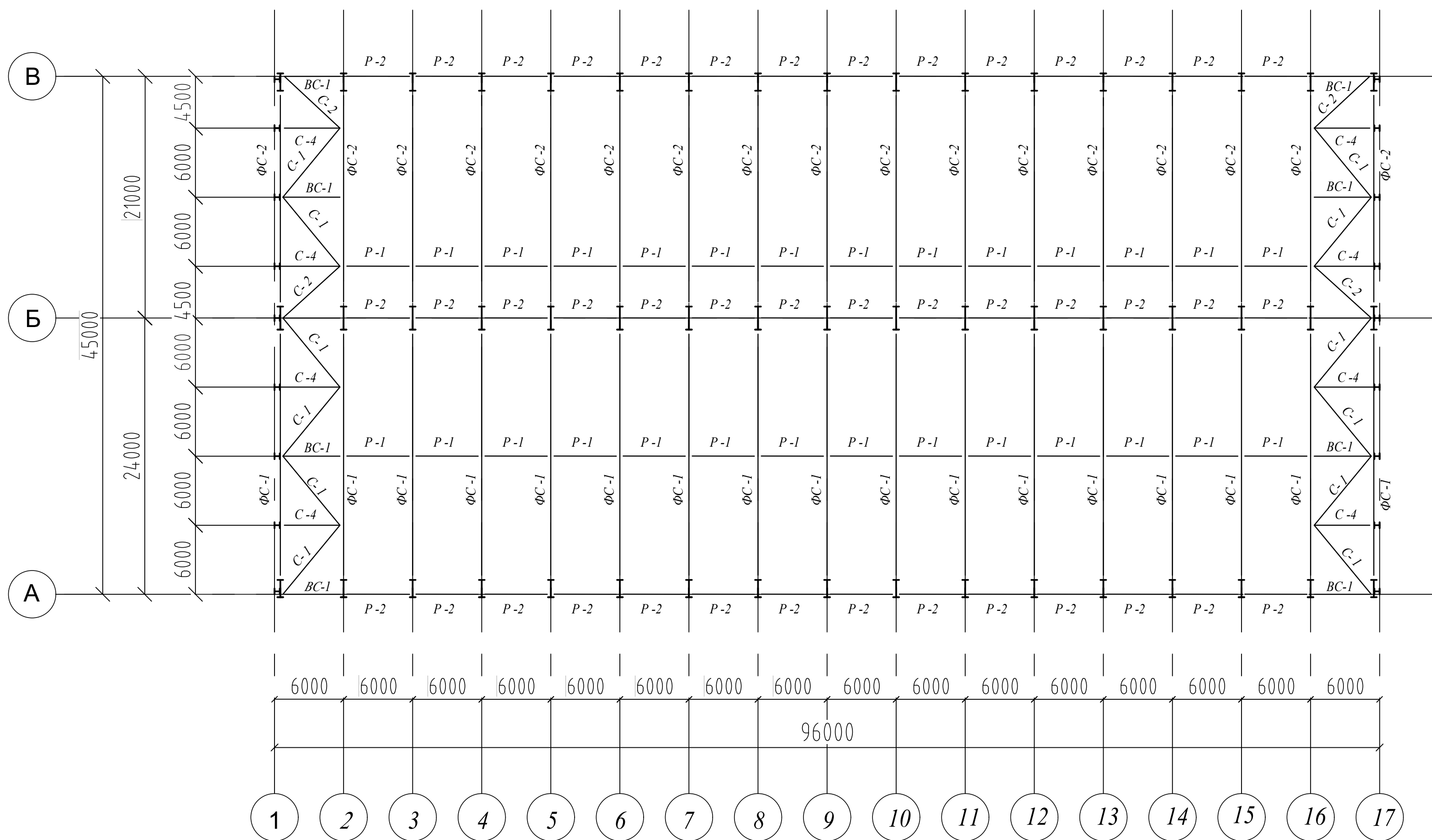
Схема расположения элементов покрытия в плоскости верхних поясов ферм
