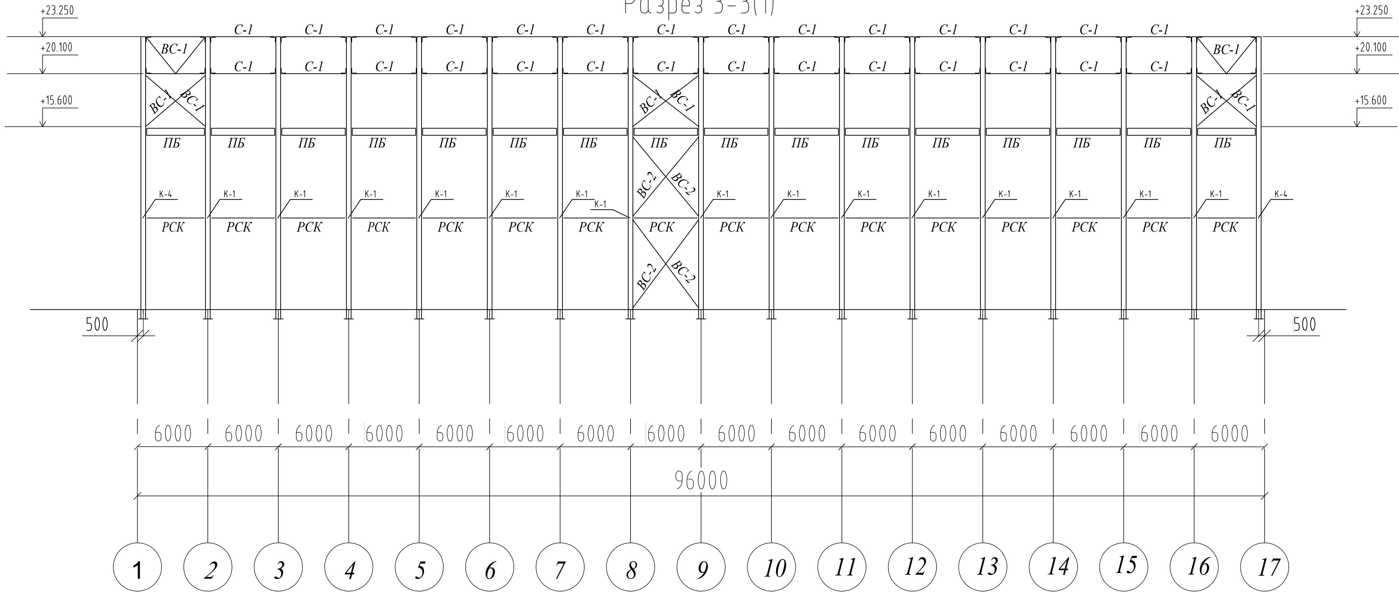
Разрез 3-3(1)
