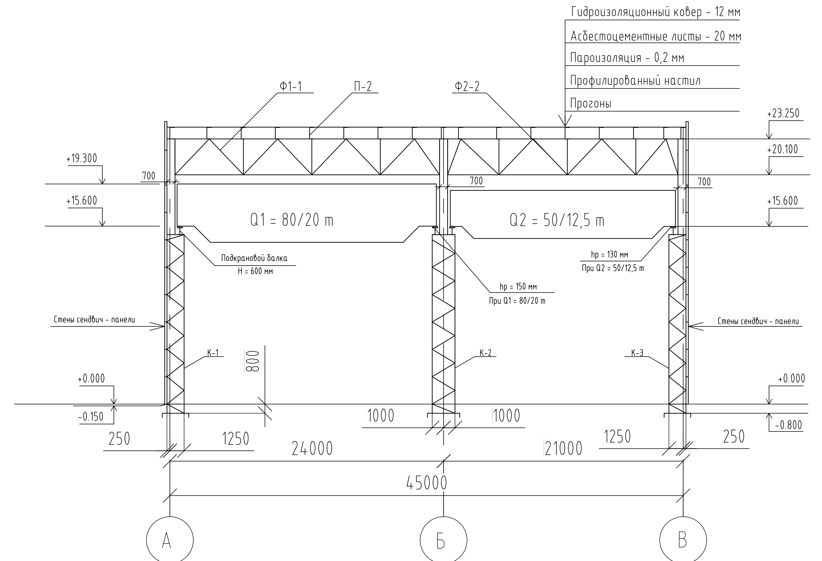
Поперечный разрез здания Разрез 1-1(1)
