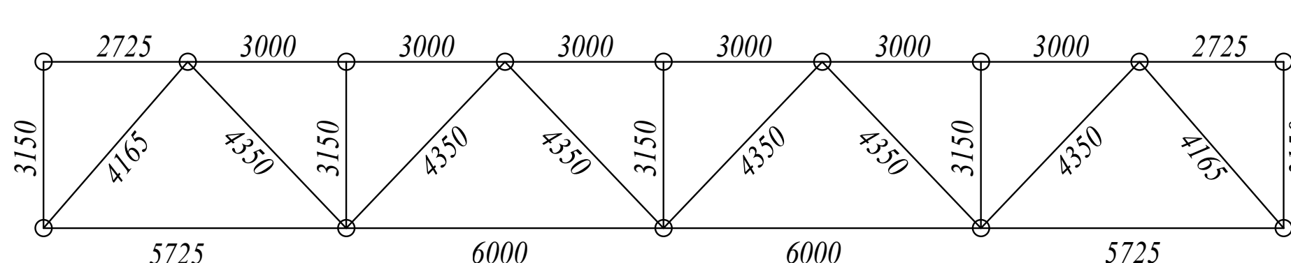
Геометрическая схема фермы Ф-1
