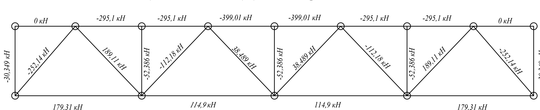
Геометрическая схема фермы Ф-1 с усилиями в кН
