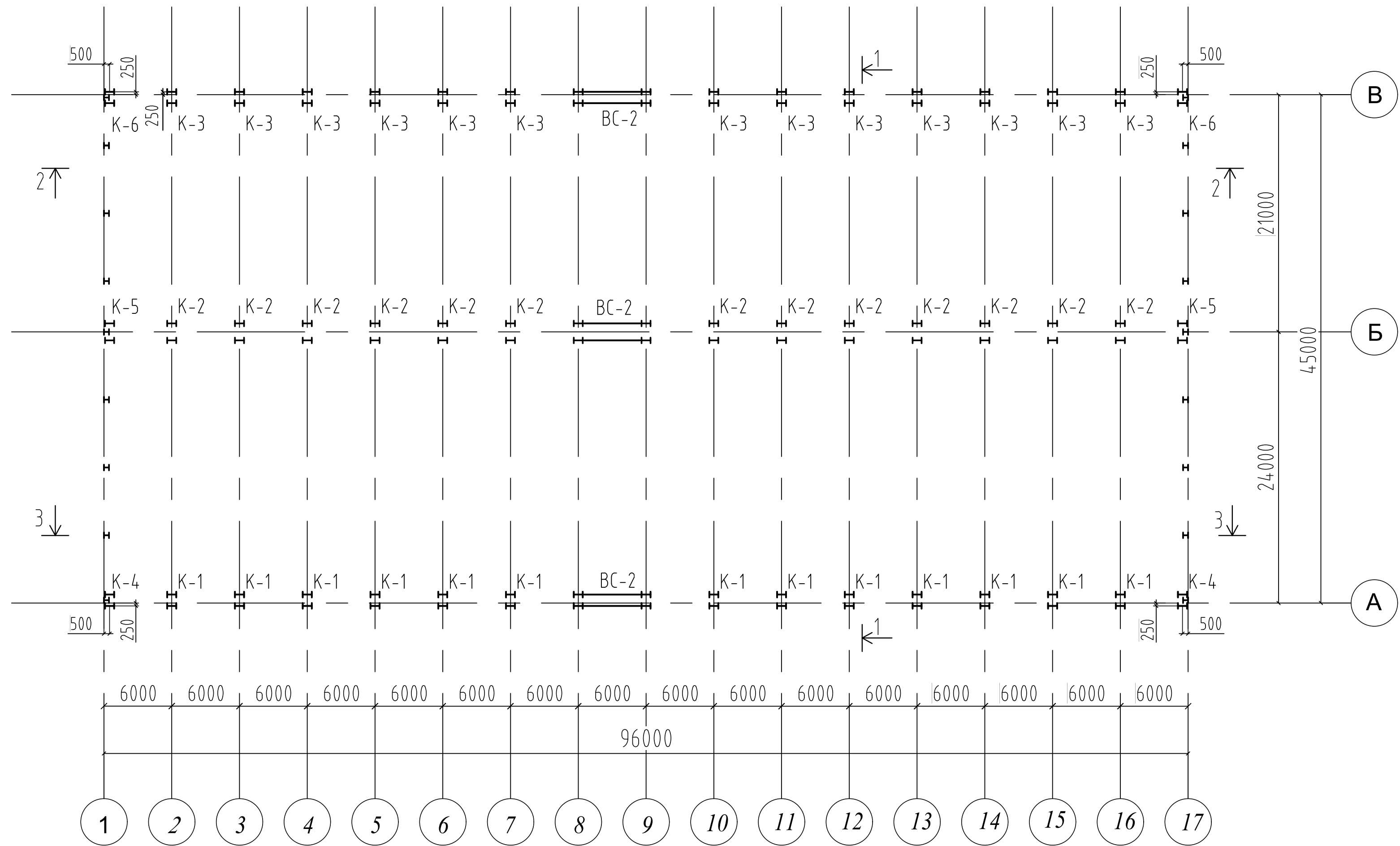
Схема расположения прогонов
